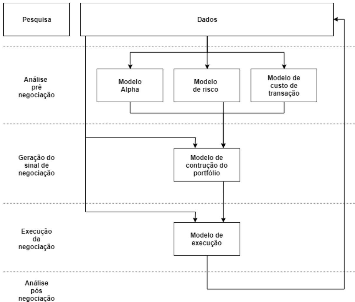
Figura 10 – Passos que ocorrem num sistema de negociação algorítmica
