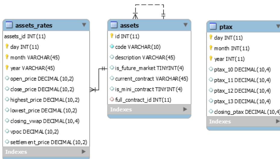
Figura 15 – Modelo relacional da base de dados interna
