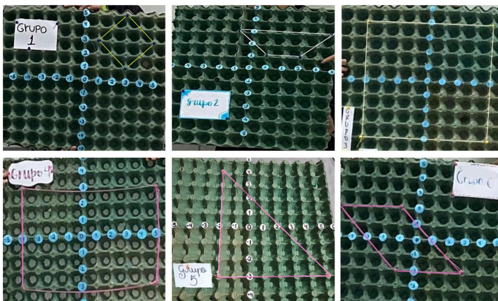
Figura 1 – Representando as figuras geométricas empregando o plano cartesiano construído.
