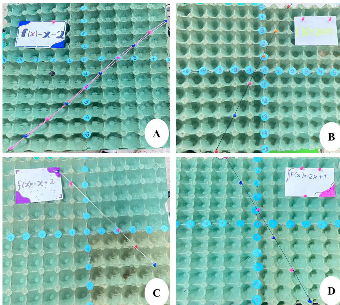
Figura 3 – Estudando função afim no Plano Cartesiano. A e B funções crescentes, C e D funções decrescentes.
