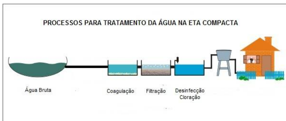
Figura 7 – Processos para tratamento da água na ETA compacta
